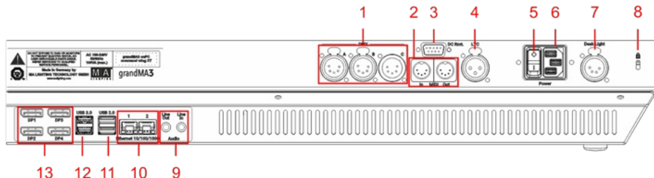
grandMA3 onPC command wing XT Rückseite
